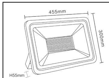
CIE-2F1-200W سری بلالی
