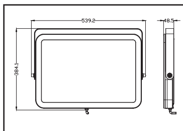
CIE-2F2-300W سری رویال
