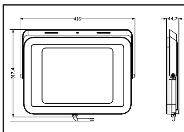
CIE-2F2-200W سری رویال
