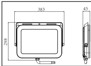
CIE-2F2-150W سری روبال
